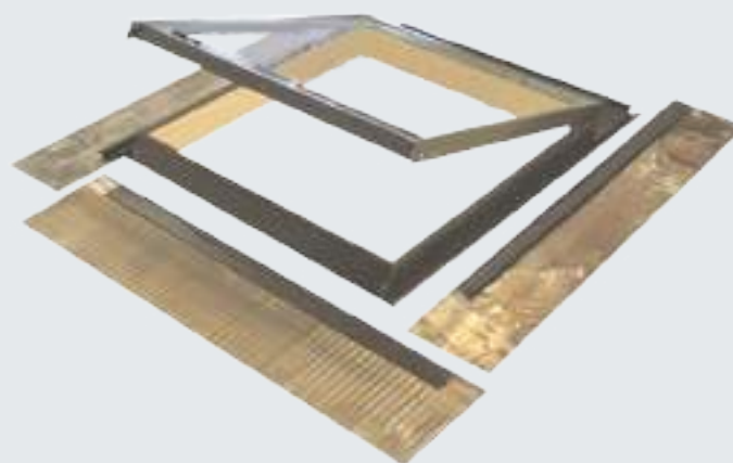
Versioni -Alluminio T. di moro -Rame -Con piombo frontale o su tre lati
